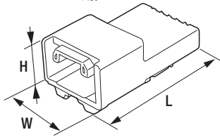
メス (オスターミナル用) B-85用
