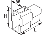
メス (オスターミナル用) B-9用
