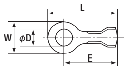
パーツ寸法
