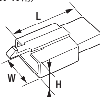
メス (オスターミナル用) B-5用
