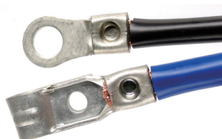
D-19N 製品圧着例
