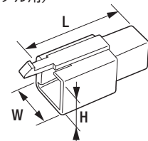
メス (オスターミナル用) B-5用
